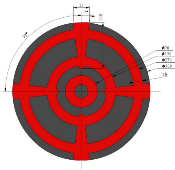
图 5-22 能量机关可激活标识示意图
