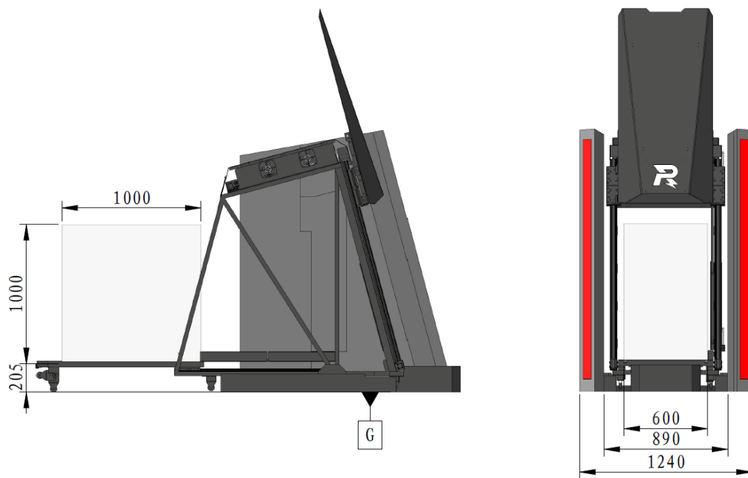
图 4-15 滑台滑出示意图
