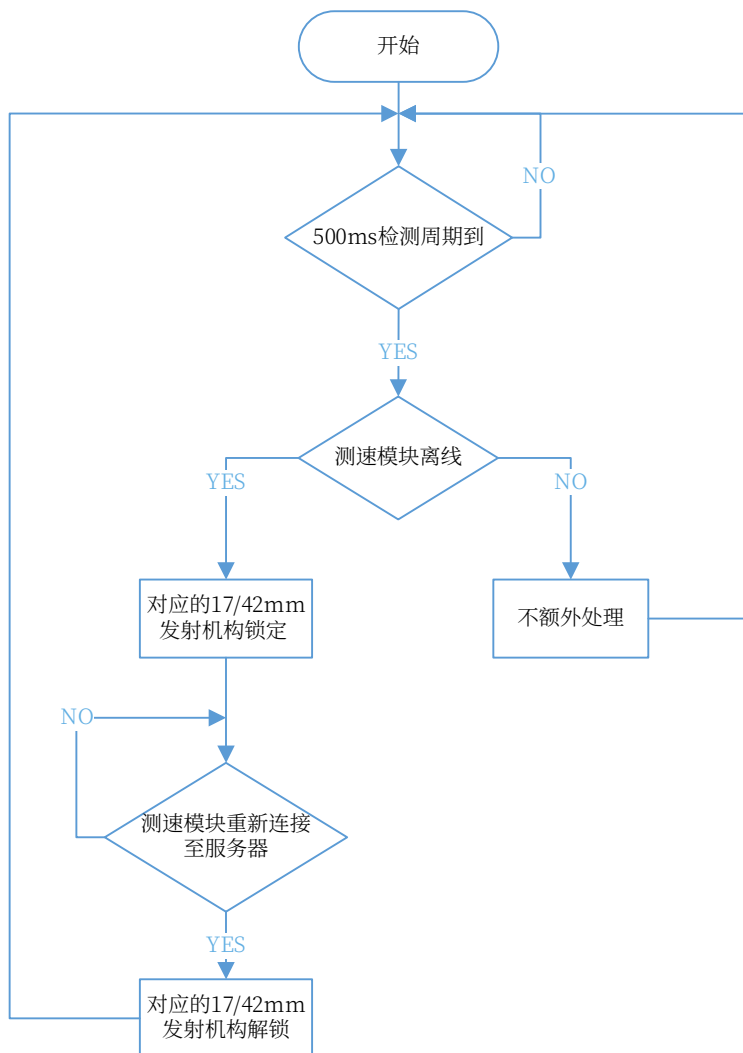
图 5-4 测速模块离线的断电机制
