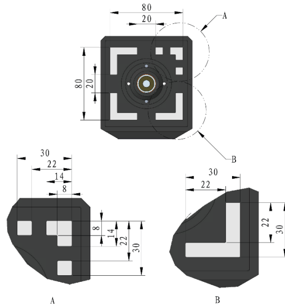
图 5-8 科技核心 MARK 灯尺寸示意图
