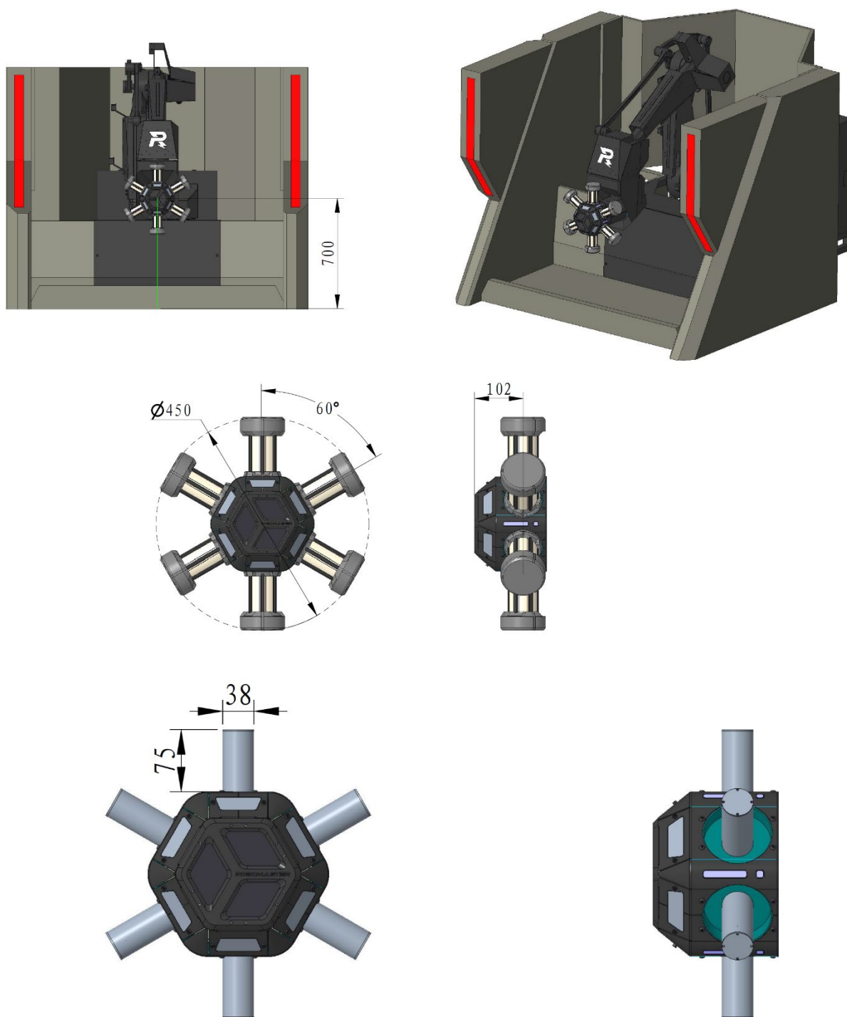
图 4-22 能量单元放置区示意图
