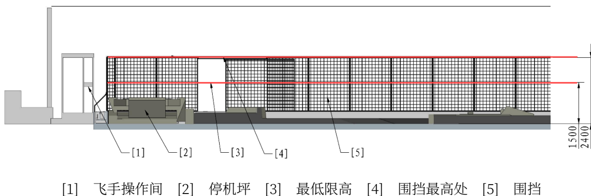
图 7-1 飞行高度限制示意图
