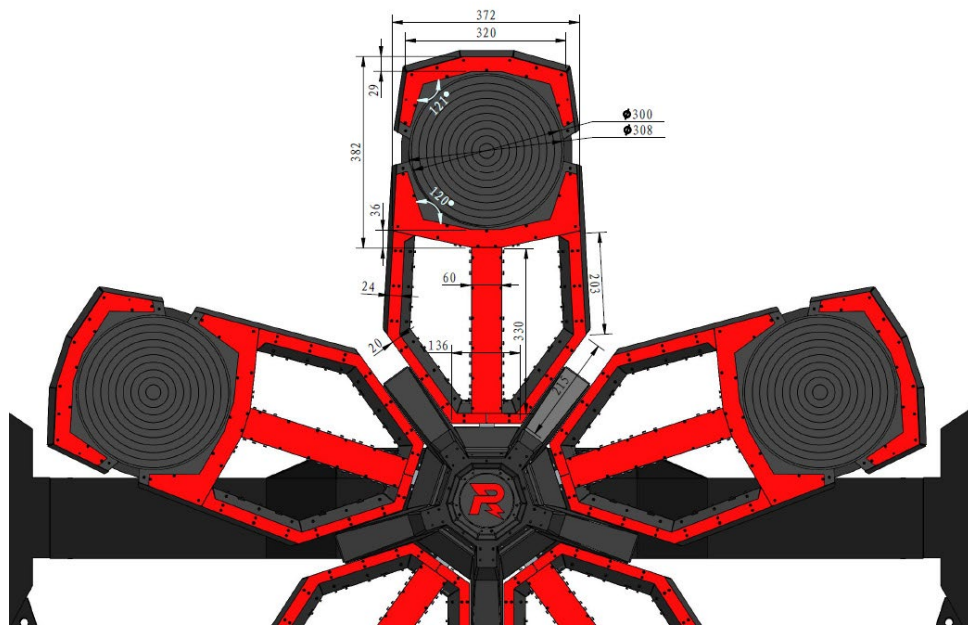
图 4-32 能量机关灯臂尺寸示意图
