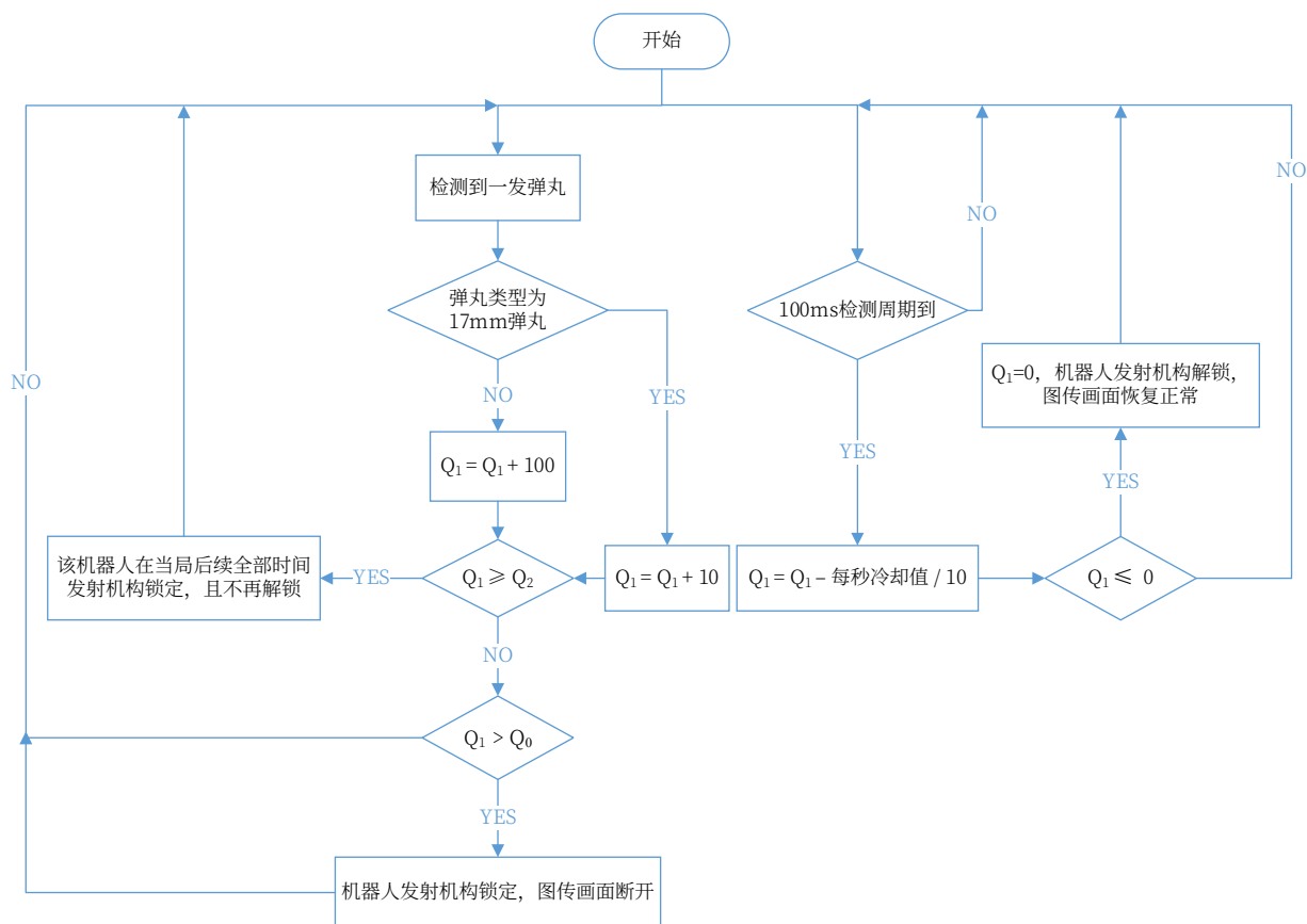
图 5-1 射击热量超限及冷却机制
