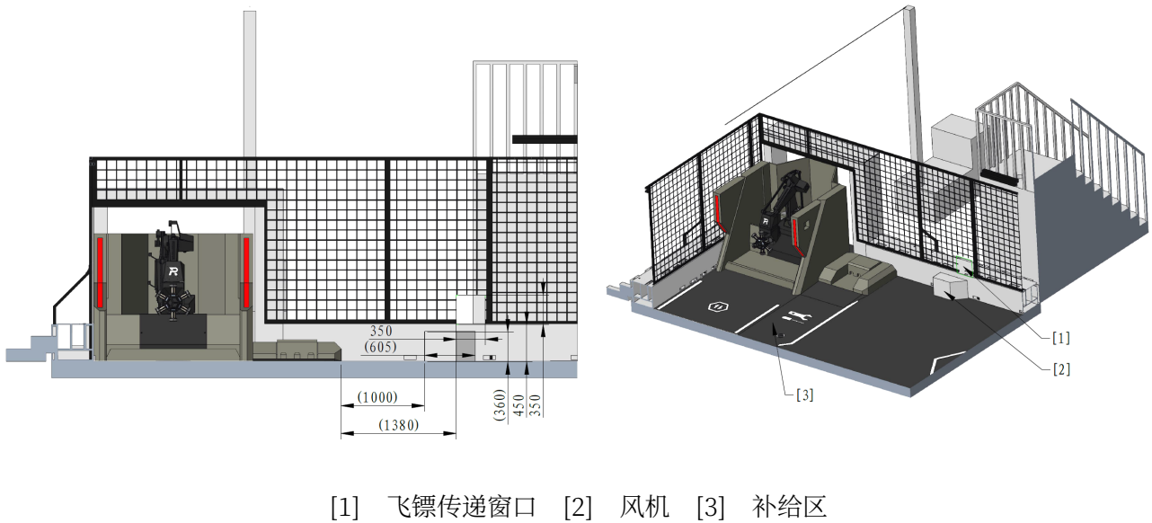
图 4-20 补给区示意图
