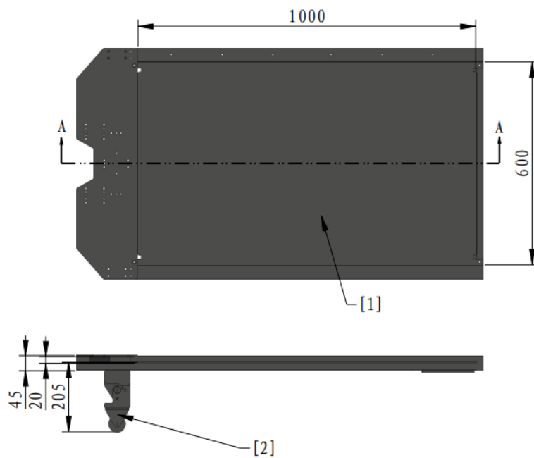
图 4-15 滑台滑出示意图
