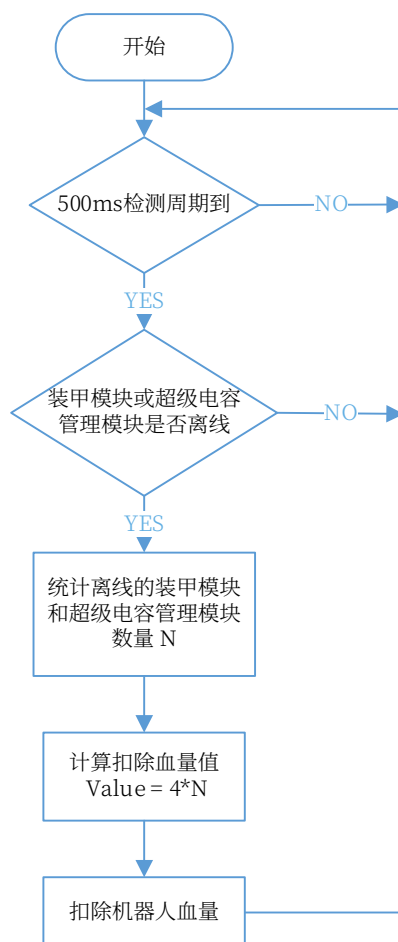
图 5-3 装甲模块和超级电容管理模块离线的扣血机制
