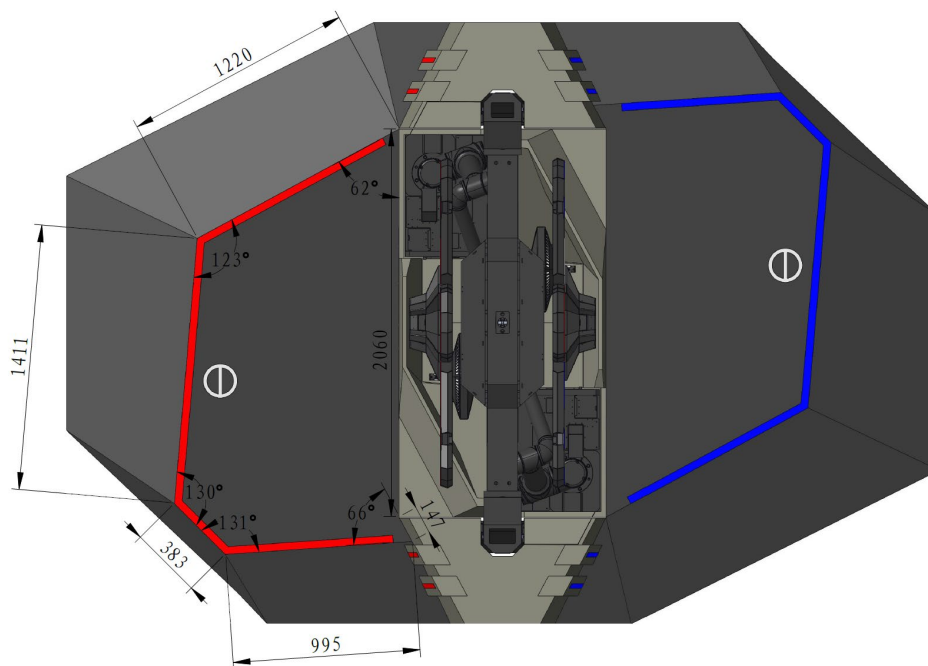
图 4-30 装配区尺寸图
