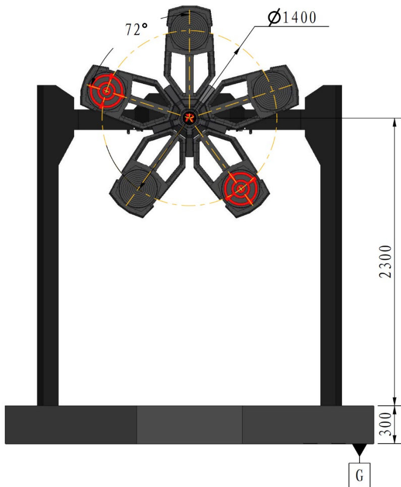
图 4-31 能量机关示意图
