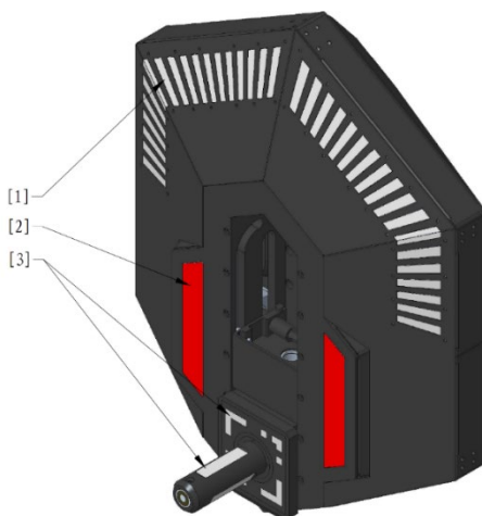
[1] 第一组灯 [2] 第二组灯 [3] 第三组灯
