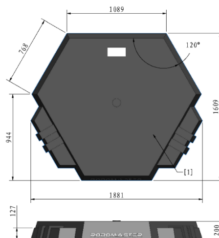
图 4-10 基地底座示意图
