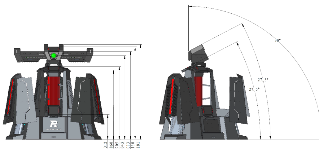
图 4-12 基地护甲展开形态尺寸图
