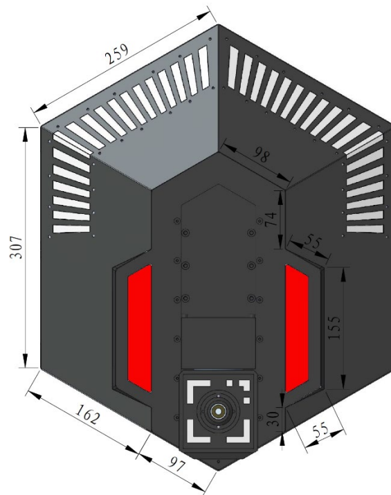
图 5-9 科技核心尺寸示意图
